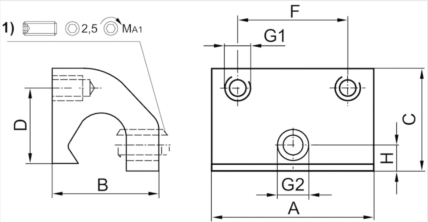
1) gwintowany trzpień zaciskowy
